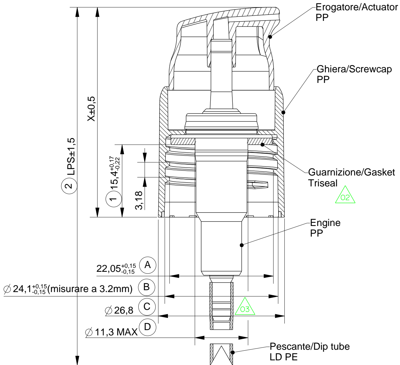
SEZIONE A-A SCALA 2:1
